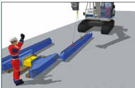
Assemblage au sol des portiques.
