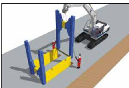
Mise en place du 2 e portique.
