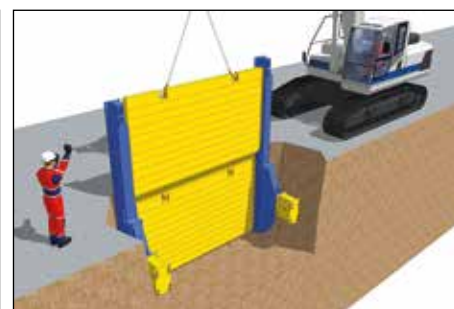
Terrasser par couches horizontales (le fond du terrassement reste constamment de niveau).
