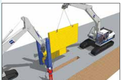
Mise en place second panneau (parallèle au 1 er panneau).
